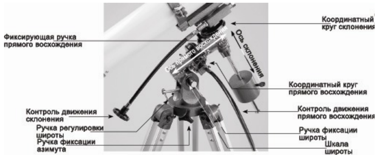
Рисунок 4. Экваториальная монтировка
