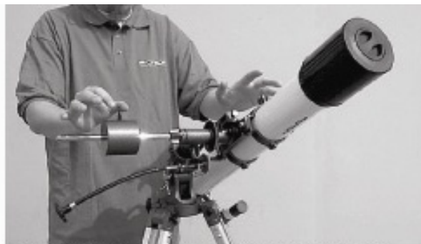
Рисунок 3б. Телескоп уравновешен вдоль оси прямого восхождения. Если отпустить руки, то стержень противовеса останется в горизонтальном положении
